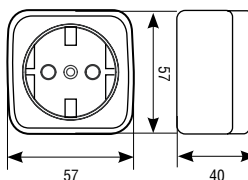
Розетка с/з
