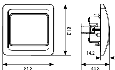
Выключатель одноклавишный
