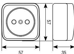
Розетка б/з
