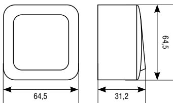
Выключатель
