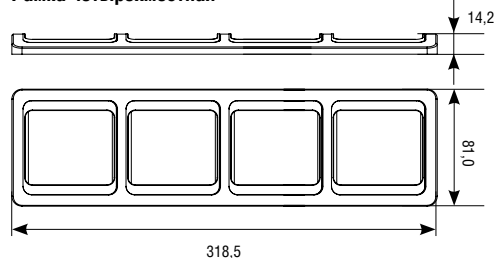
Рамка четырехместная
