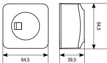
Розетка компьютерная
