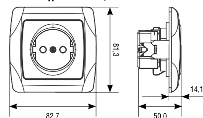
Розетка одноместная с/з
