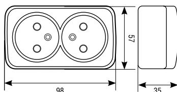
Розетка двухместная б/з
