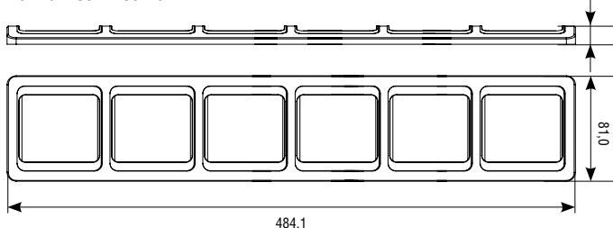
Рамка шестиместная
