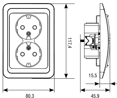
Рамка двухместная
