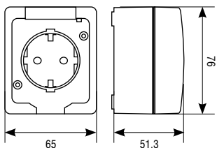
Розетка
